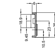
Allgemeine Vermaßung
