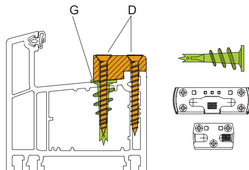
Alternative 2 / Bild 2 Montagesituation z.B. GKM Dübel Fischer
