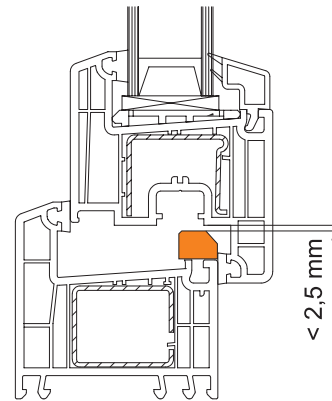
Bild 1: Position des Auflaufes, Luft zwischen Auflauf und Flügelkante
