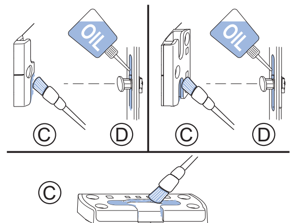
Schmierstellen
