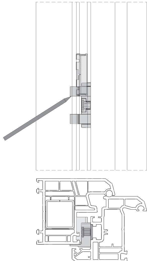
Bild 2 : Positionsmarkierung Rahmenteil
