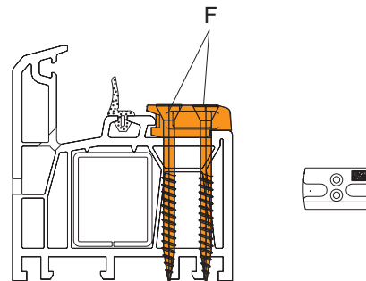
Alternative 3 / Bild 3 Montagesituation Nut (Trocal)
