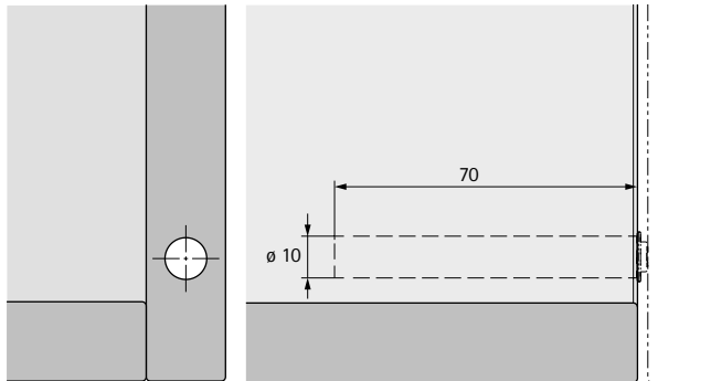
Bohrbild für Langhub, vorliegende Tür
