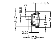
Allgemeine Vermaßung
