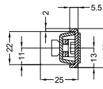
Fräsmaße
