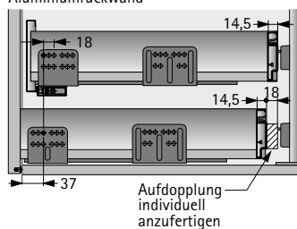
Aluminiumrückwand
