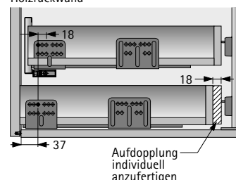
Holzrückwand
