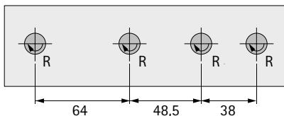
Bohrbild
