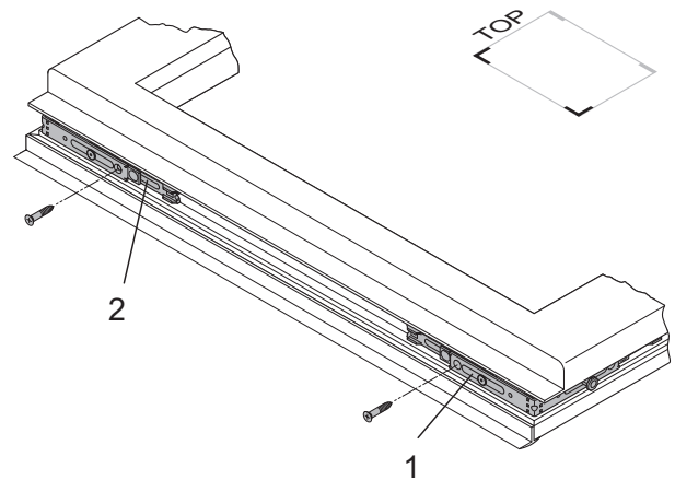
Eckumlenkungen E1
