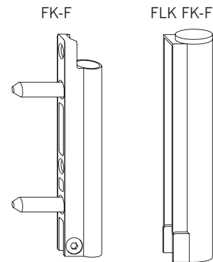
Flügelager mit Justierschraube zur Regulierung der Drehhemmung
