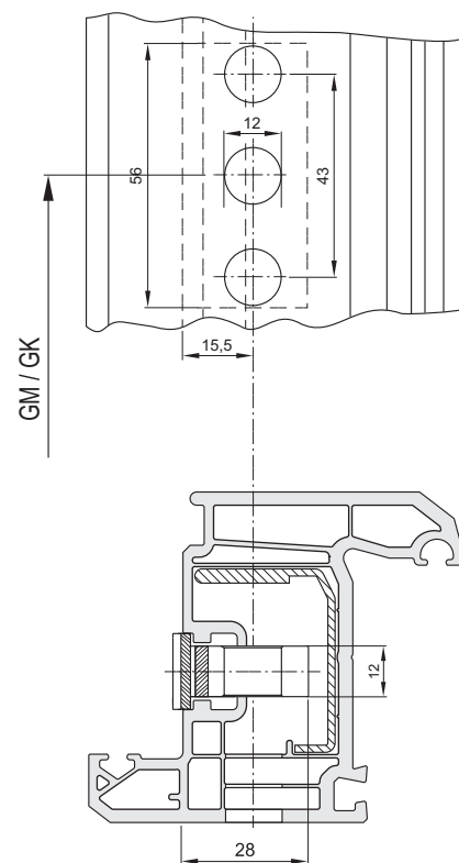
Maßzeichnung "Getriebebeschloss"
