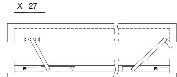
B-7-5: Einbauzeichnung Zusatzschere ZSRE (für Beschlagausführung "Kipp vor Dreh")
