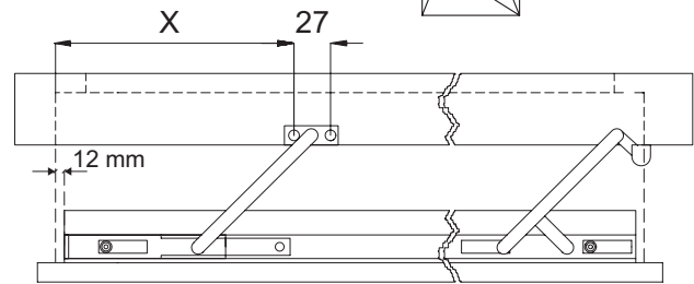
B-7-4: Einbauzeichnung Zusatzschere ZSR (X bezogen auf Rahmenfalzkante)
