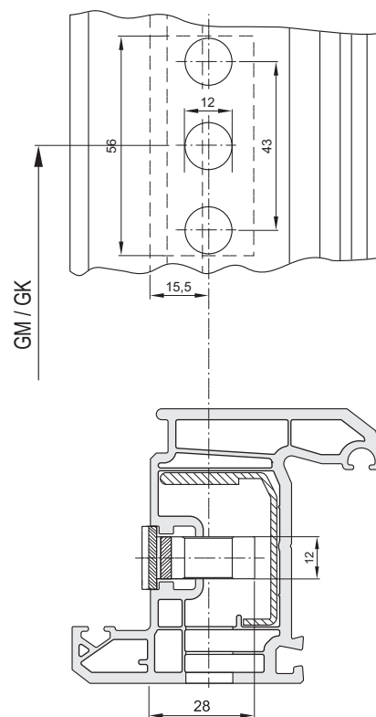
Maßzeichnung "Getriebebeschloss"
