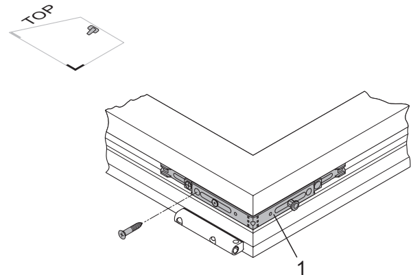
Eckumlenkung E1
