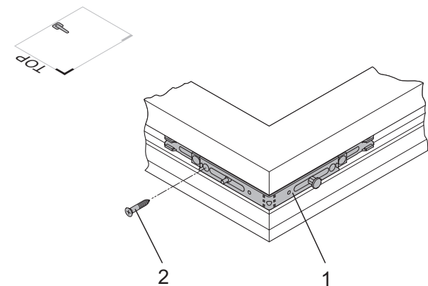
Eckumlenkung E2
