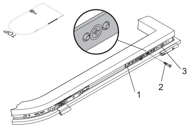
Mittenverriegelung MK
