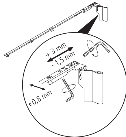
Schere - Atelierfenster
