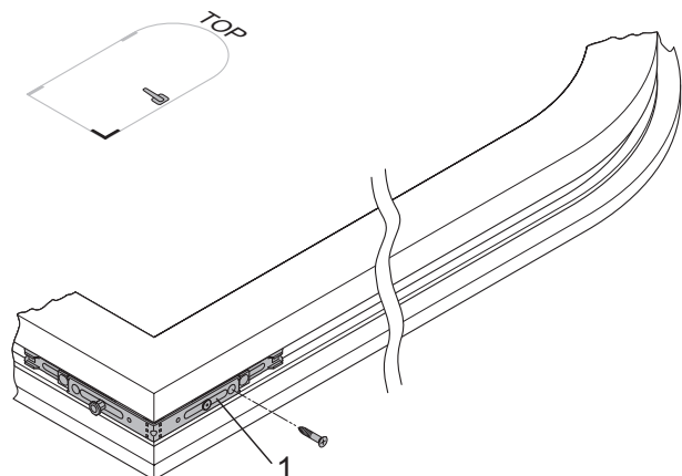
Eckumlenkung E1
