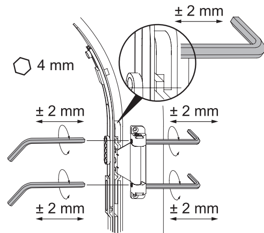
Schere - Rundbogenfenster
