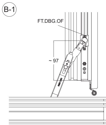
B-10-4: Drehbegrenzer DBG
