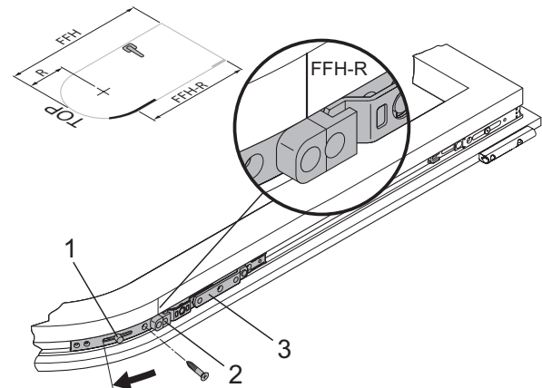
Schere GRT.SWR
