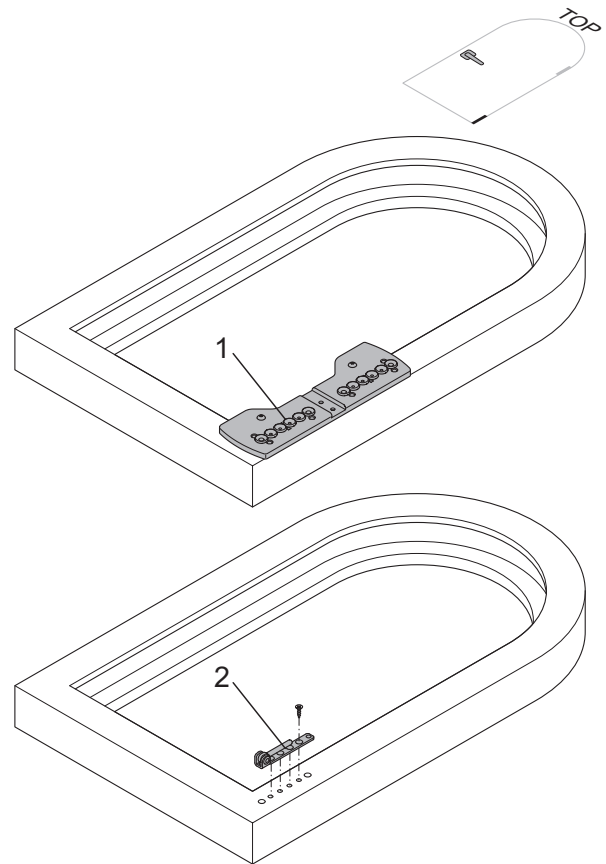
Ecklager / Bohrlehre
