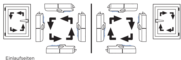
Schließblechposition "konstanter Griffsitz"
