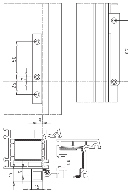
B-10-2: Bohrbild Öffnungsbegrenzer OBV
