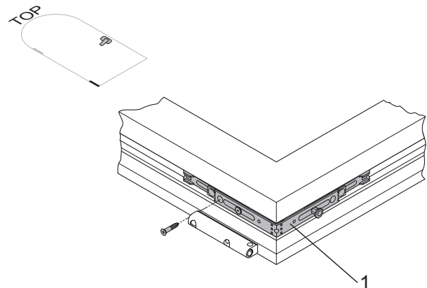
Eckumlenkung E1
