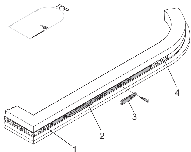
Getriebschiene GAM/GAK
